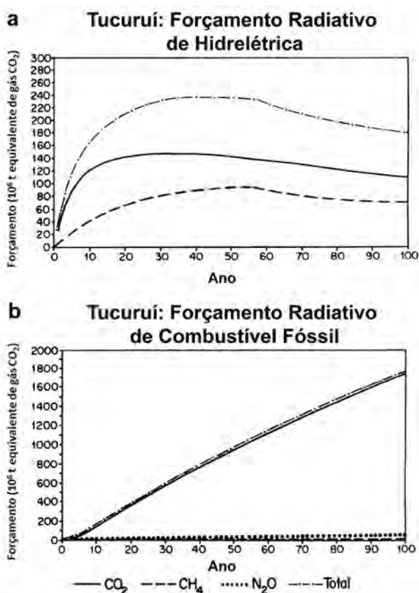
Figura 5. Tucuruí: forçamento radiativo das cargas atmosféricas de gases de efeito estufa (A) a partir do projeto da hidrelétrica, (B) a partir de combustíveis fósseis deslocados por Tucuruí. O centro de gravidade da curva de forçamento radiativo total é no ano 52 para as emissões de hidrelétricas e no ano 67 para emissões a partir de combustíveis fósseis, uma diferença de 15 anos.
