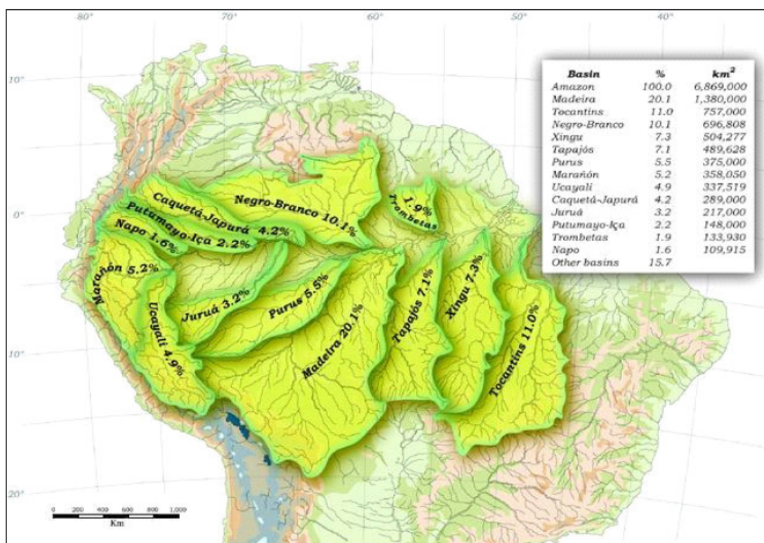
FIGURA B.II. 3 - Mapa esquemático mostrando as principais bacias tributárias do sistema Solimões/Amazonas. (EIA-Tomo B 1/8, p. II-6)
