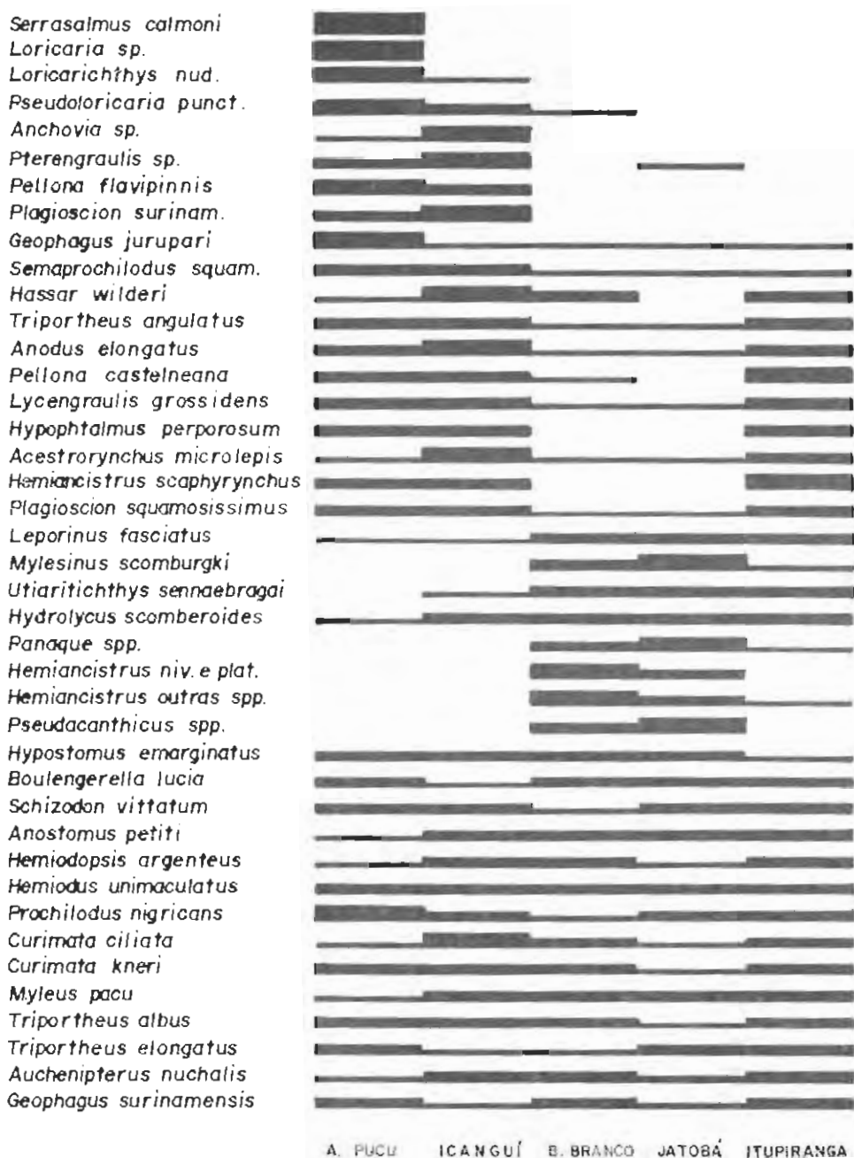
Fig. 5. Distribuição espacial das espécies mais significativas na calha principal do baixo Tocantins entre Cametá e Marabá.
